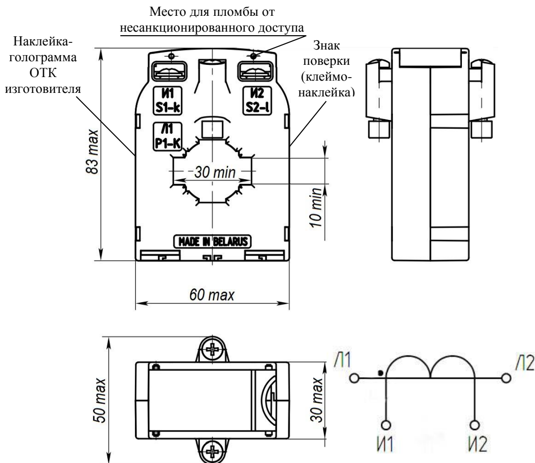
Рис. А.1 Габаритный чертеж, схема электрическая принципиальная
